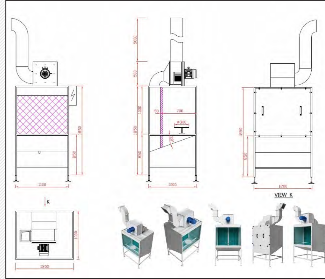
Spray Cabinet SKU: GSI-001
